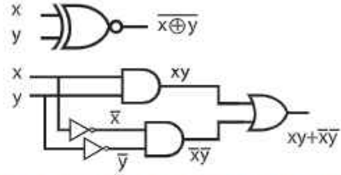
চিত্র 3.13: XNOR গেটের সত্যক সারণি, প্রতীক এবং লজিক
